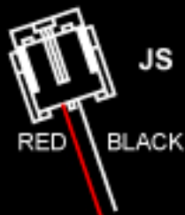
JST02C01(JST EHR-2)
